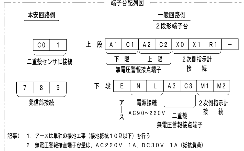
端子台配列図
